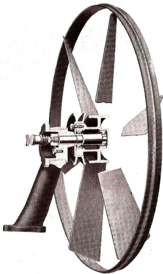
Radiator Fan
