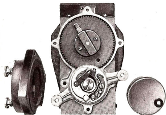
Magneto
