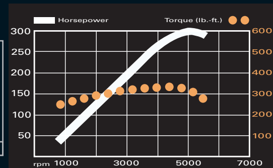
5.3L Vortec 5300 V8
