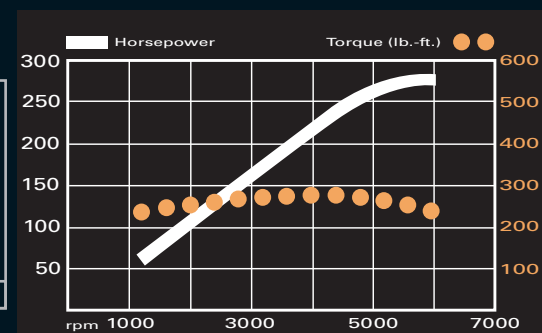
4.2L Vortec 4200 I-6
