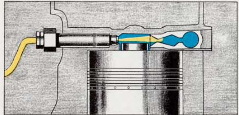
"Energy Cell"
