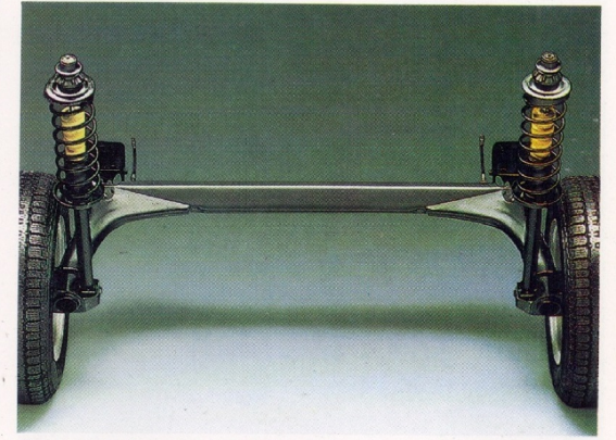
Eje trasero. - Seguridad de marcha y gran confort. Sus conjuntos de goma y metal reaccionan con suavidad en las rectas, en las curvas oponen una firme resistencia a las fuerzas laterales.
