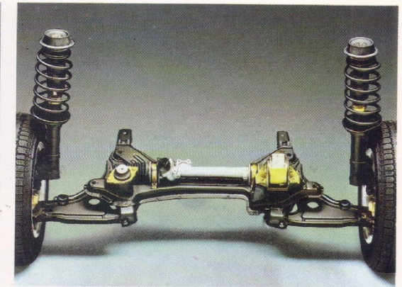
Eje delantero. - Sinónimo de estabilidad de marcha, elevado confort en ruta, facilidad de manejo.
