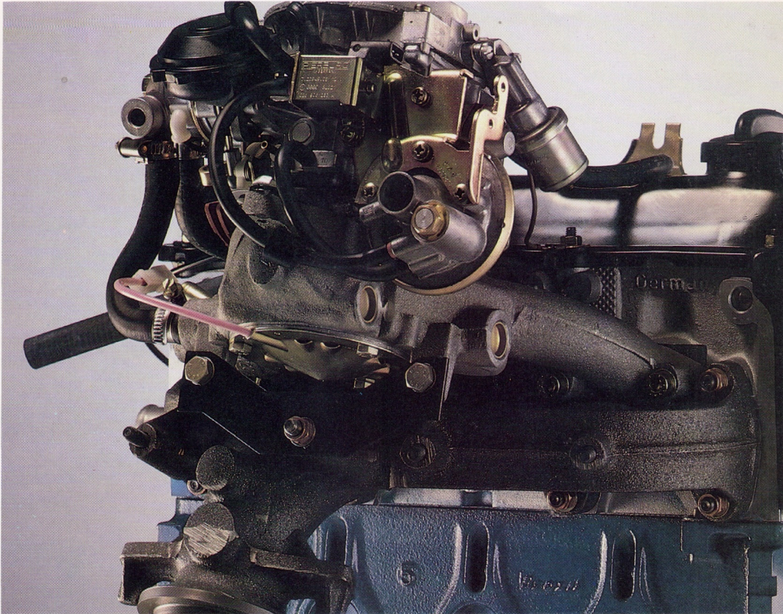
Motor de 1800 c.c. - Notable por su suave funcionamiento y el despliegue de su fuerza.
