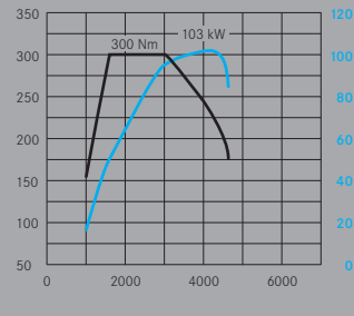
B 200 CDI
