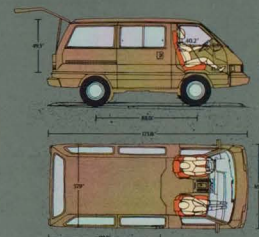
CARGO VAN DIMENSIONS
