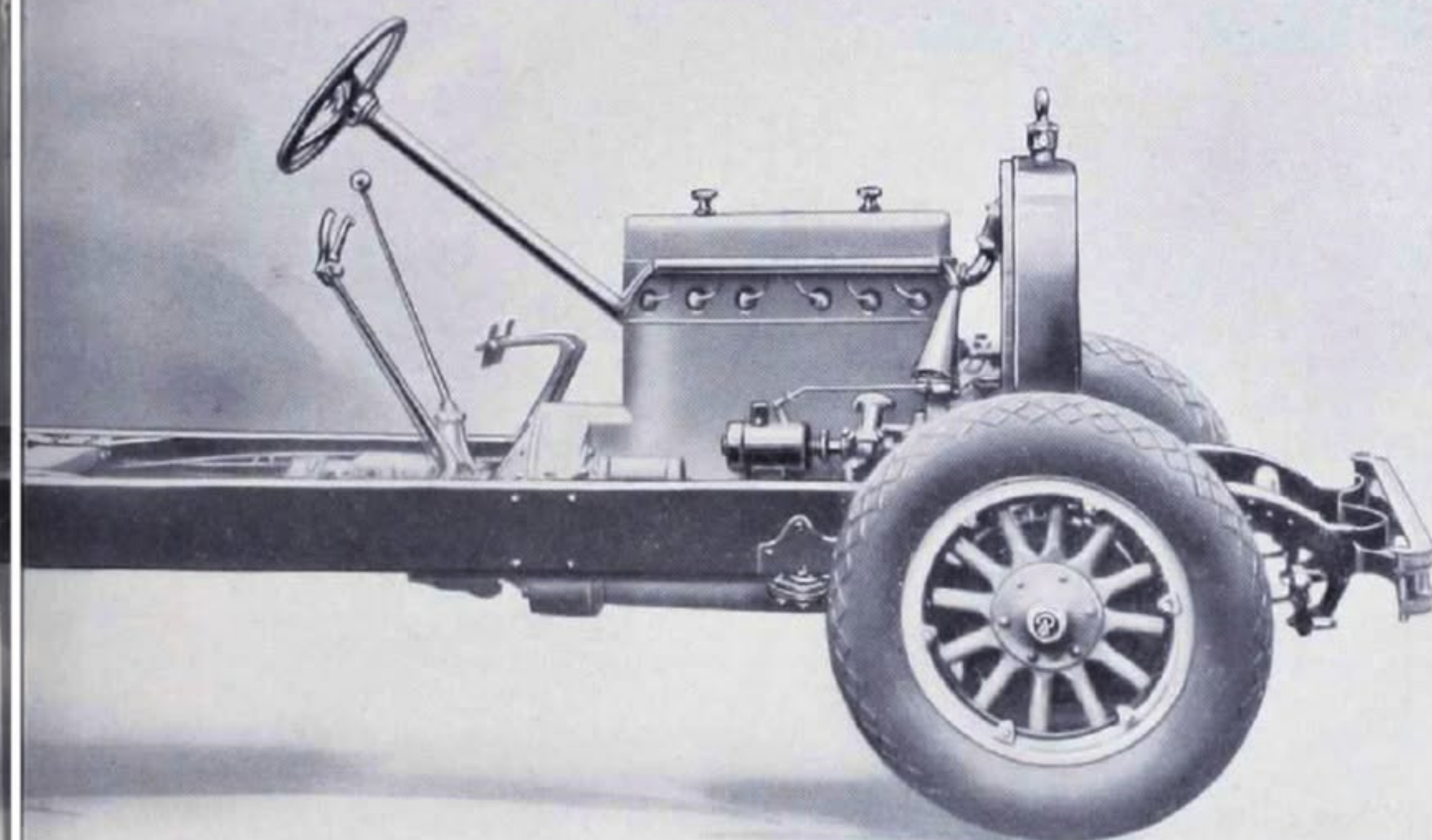
DU PONT CHASSIS
